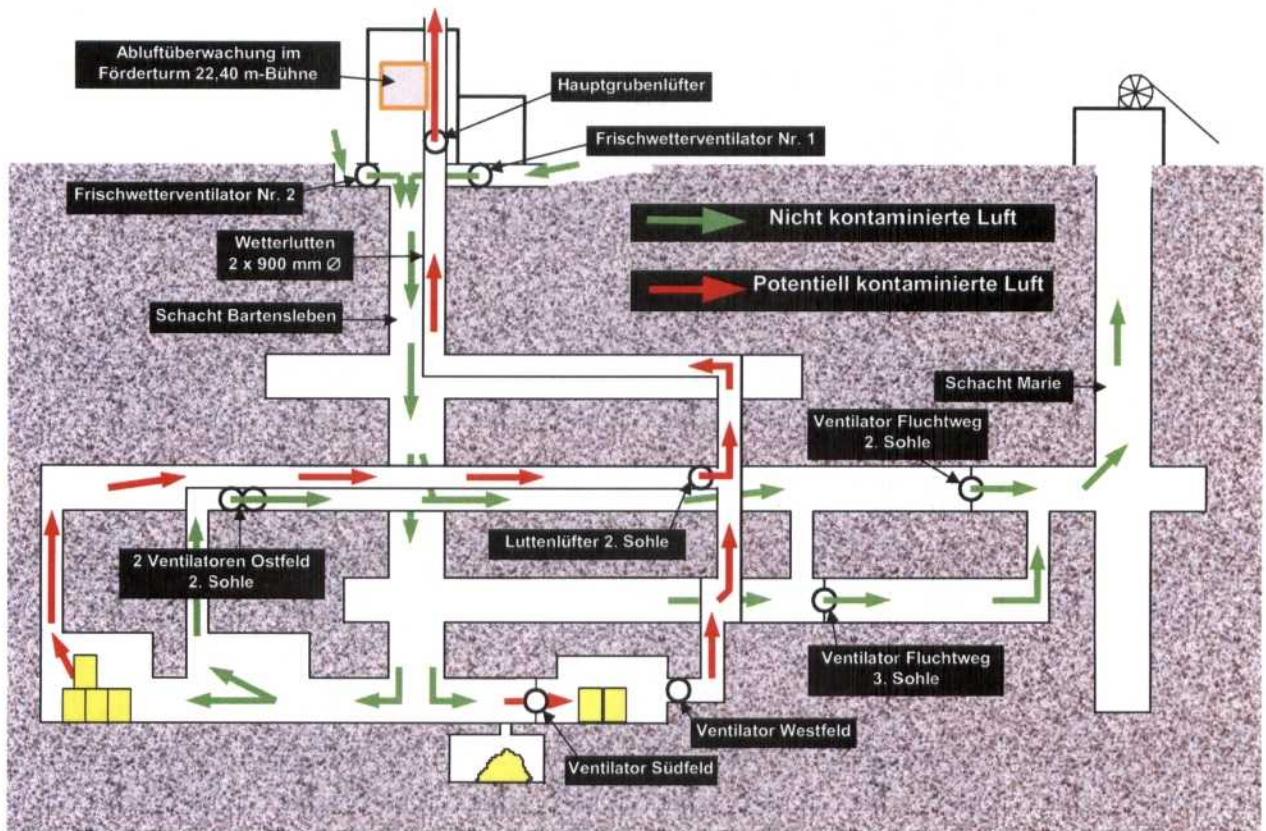
Abb. 2.1: Schematische Darstellung der Bewetterung der Einlagerungsbereiche (außer Flächen 5)
