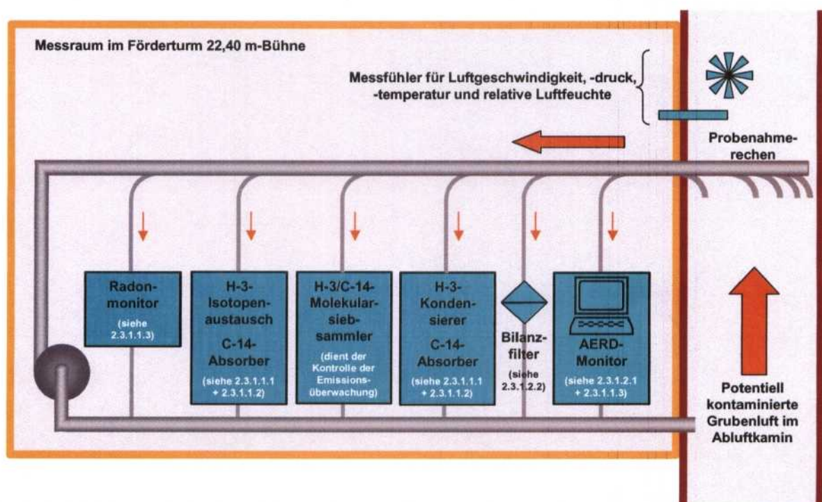
Abb. 2.2: Schematische Darstellung der Abluftprobenahme und -messung
