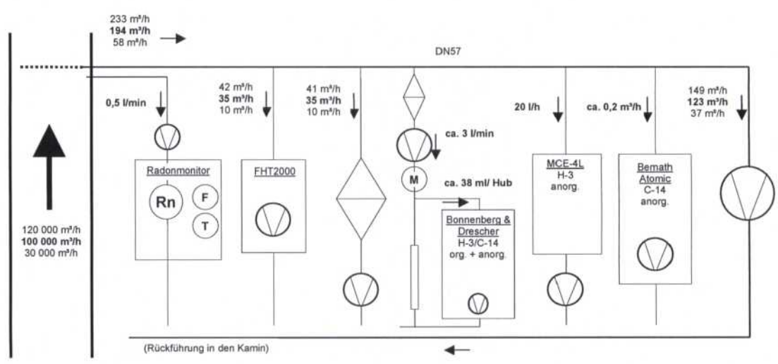
Abbildung: Schematische Darstellung der Abwetterüberwachung an der Messstelle Kamin Schacht Bartensleben
