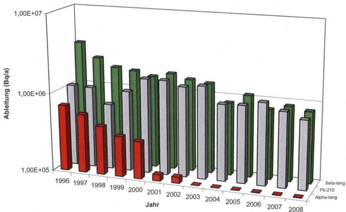
Abbildung 3.1.6 : Radioaktive Aerosole (Beta-lang, Pb-210, Alpha-lang)
